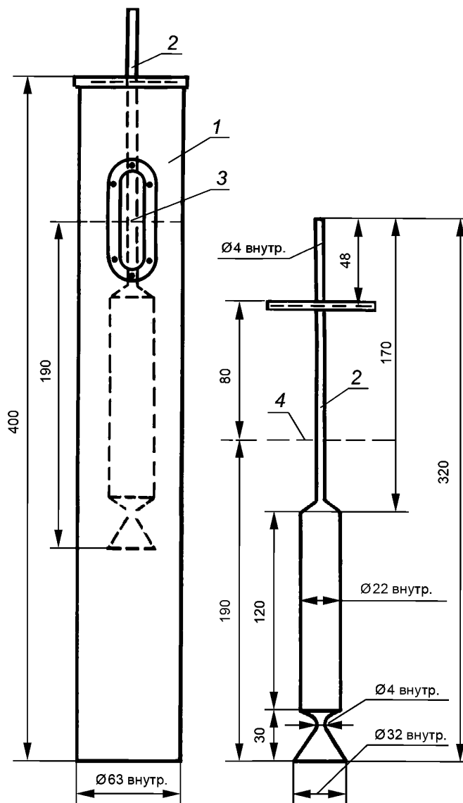
1 — цилиндр; 2 — пипетка; 3 — метка ( 1000 \text{ см}^3 ); 4 — уровень суспензии в цилиндре
